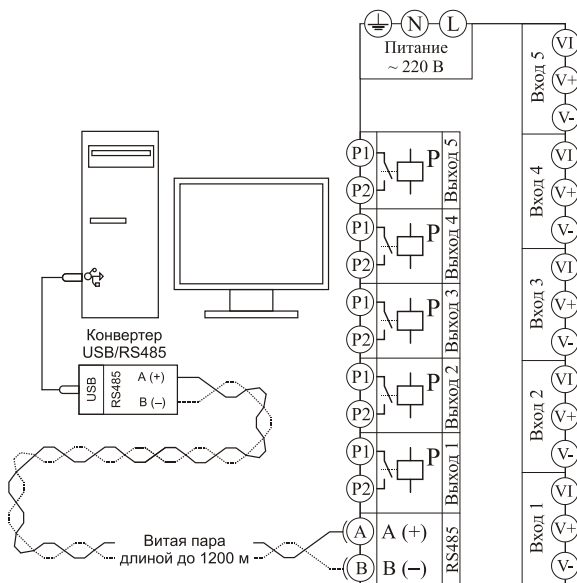
Рис 1. Подключение к компьютеру (для приборов с интерфейсом)
